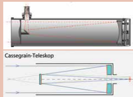
Şekil 2a ve 2b : "Newtonian" ve "Cassegrain" tipi yansıtıcı teleskoplarının çalışma prensipleri
