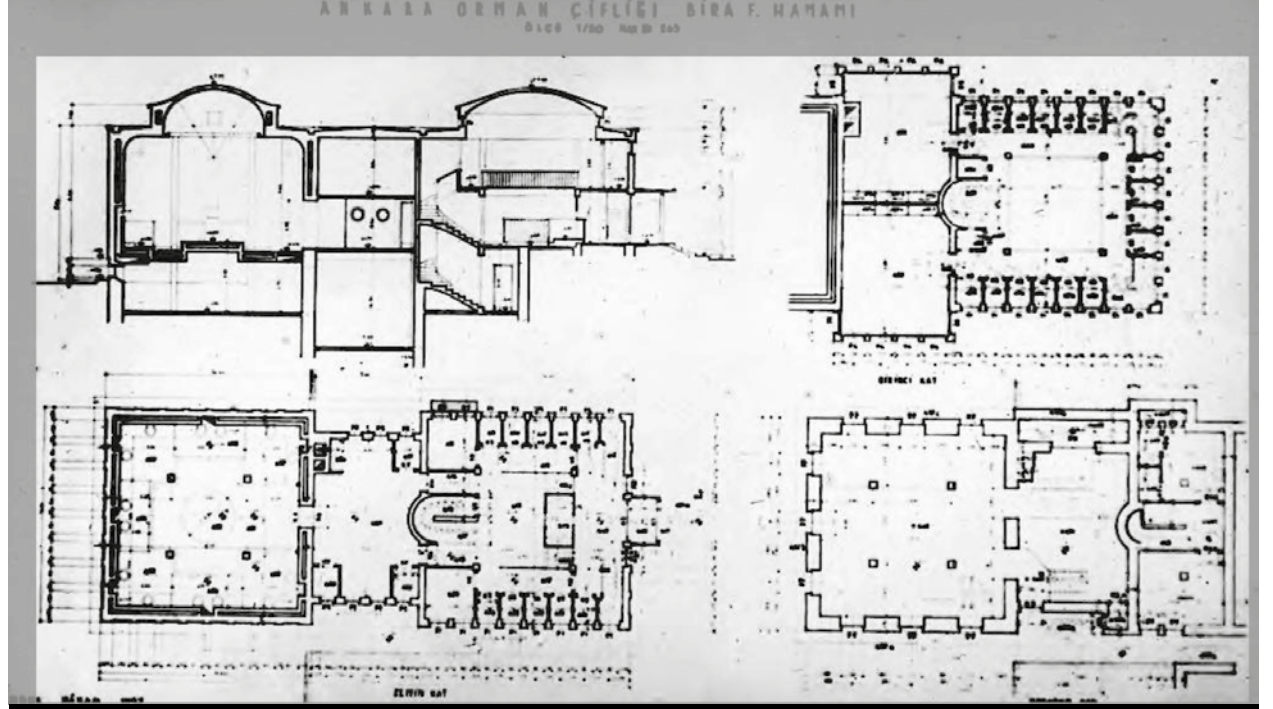
AOÇ Hamamı kat planları ve kesit Kaynak: Büşra Kul (2012), Conservation Proposal of An Early Republic Period Building: Atatürk Orman Çiftliği Hamamı. Basılmamış Yüksek Lisans Tezi, ODTÜ Restorasyon Bölümü
